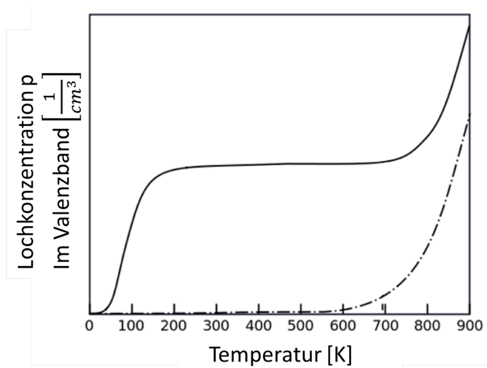
Abbildung 4: Lochkonzentrationen im Valenzband in Abhängigkeit von der Temperatur
