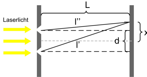
Abb. 2: Skizze zum Doppelspalt-Experiment
