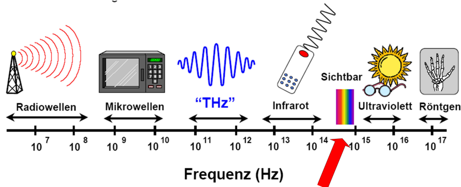
Abb. 1: Spektrum elektromagnetischer Strahlung
