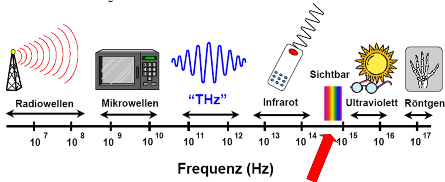
Abb. 1: Spektrum elektromagnetischer Strahlung
