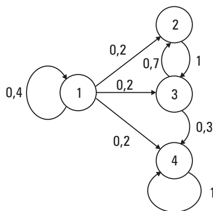
Abbildung 1: Übergangsgraph.
