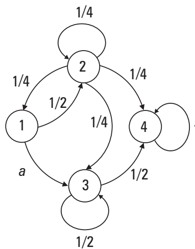
Abbildung 2: Übergangsgraph.
