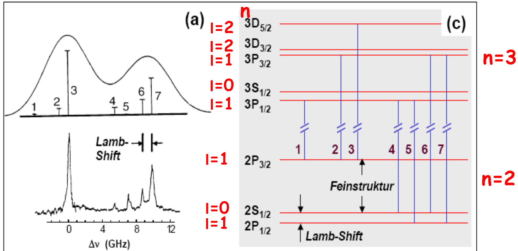
Abbildung 4.1: Feinstruktur der Balmer-Linie H_\alpha gemessen mit (a) hochauflösender Spektroskopie und (b) mit höchstaflösender Laser-Spektroskopie. (c) Verfeinertes Termschema des Wasserstoffs. Die erlaubten Übergänge werden durch die Auswahlregeln bestimmt, die wir erst später diskutieren werden.
