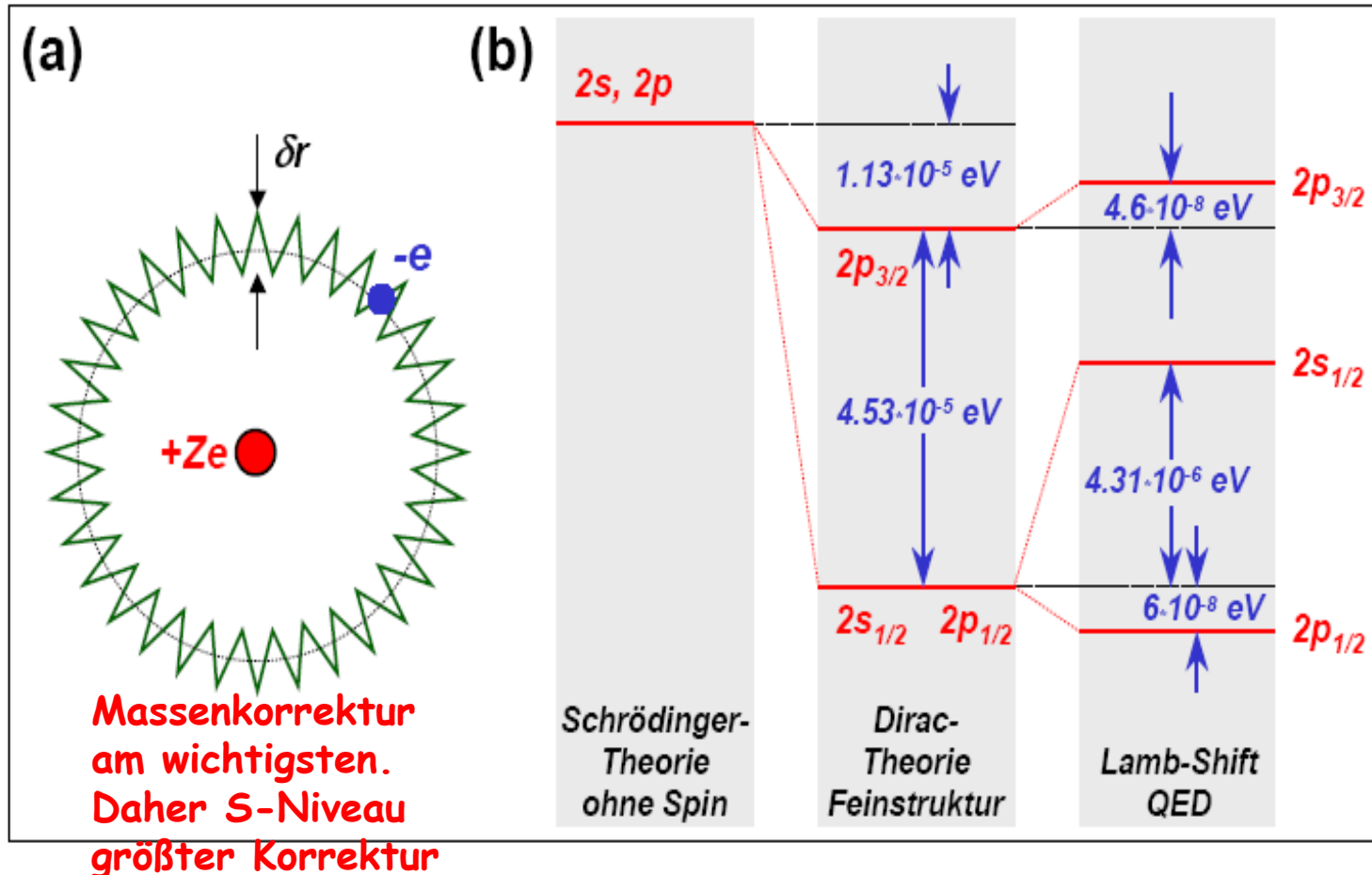
Abbildung 4.6: (a) Zur Veranschaulichung der Zitterbewegung eines Elektrons aufgrund der Emission und Absorption von virtuellen Photonen. (b) Feinstruktur und Lamb-Verschiebung beim Wasserstoffniveau mit n = 2 .
