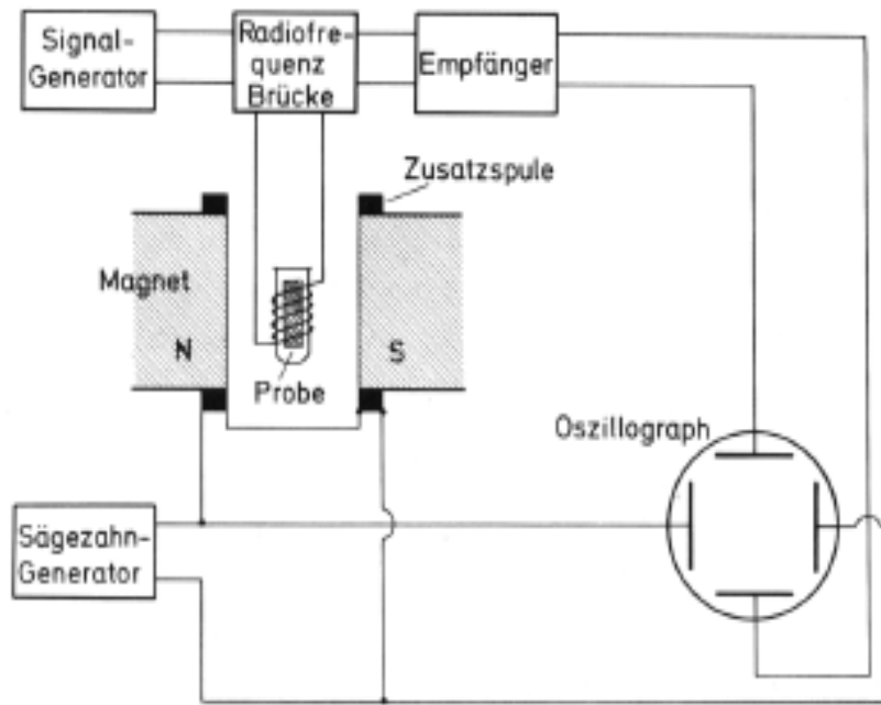
Abb. 20.18. Schema einer einfachen Kernspin-Resonanz-Apparatur. Die Probe befindet sich im Reagenzglas zwischen den Polschuhen eines homogenen Magneten. Das hochfrequente B_1 -Feld wird über eine Brücke und eine Induktionsspule eingestrahlt. Zum besseren Nachweis der Resonanz kann das B_0 -Feld durch eine Zusatzspule moduliert werden
