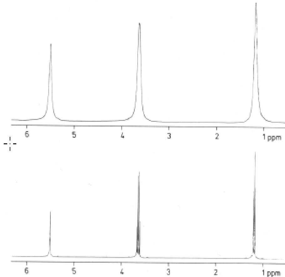
Abb. 20.20. Kernspinresonanz von Aethylalkohol, C_2H_5OH . Aufgetragen ist die Signalintensität am Empfänger als Funktion der Übergangsfrequenz. Diese ist in ppm (parts per million) relativ zu einem geeigneten Standard gemessen. Man sieht im oberen Teilbild 3 Signale mit dem Flächenverhältnis 1:2:3. Sie gehören zu den Protonenspins in der OH-, der CH_2 - und der CH_3 -Gruppe mit 1, 2 und 3 Protonen. Durch die unterschiedliche chemische Bindung unterscheiden sich die Resonanzfrequenzen der Protonen in den verschiedenen Bindungen um einige ppm. – Im unteren Teilbild ist dasselbe Spektrum mit höherer Auflösung gemessen. Das CH_2 -Signal ist jetzt durch indirekte Kernspin-Wechselwirkung mit den Protonen der CH_3 -Gruppe in ein Quartett aufgespalten, das CH_3 -Signal durch indirekte Wechselwirkung mit den CH_2 -Protonen in ein Triplett. – Die Protonen der OH-Gruppe werden rasch zwischen verschiedenen Molekülen ausgetauscht. Dadurch wird indirekte Wechselwirkung ausgemittelt und die Linie bleibt einfach
