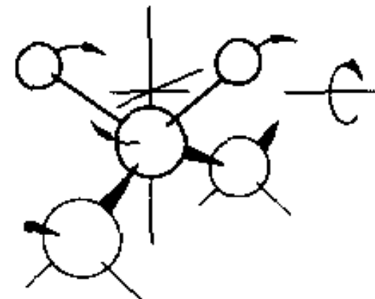
c) wagging: 1305\text{ cm}^{-1}
