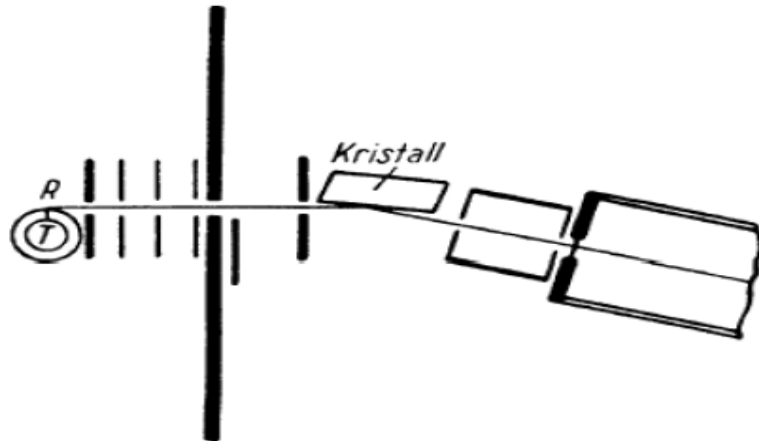
Versuchsanordnung von Compton (Molybdäncathode T, Streuung am Graphit R, Kristall als Wellenlängendetektor)
