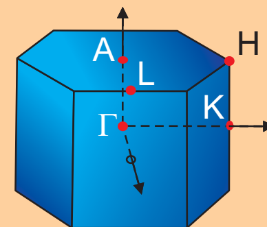
1. Brillouin-Zone des hexagonalen Gitters
