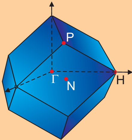
1. Brillouin-Zone des kubisch-raumzentrierten Gitters (bcc)
