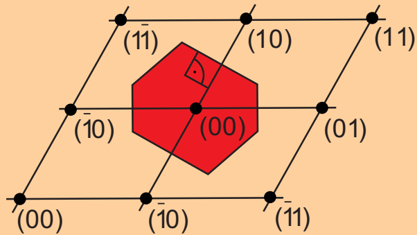
1. Brillouin-Zone des ebenen schiefwinkligen Gitters
