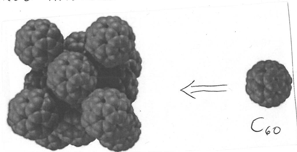
van der Waal - kräfte
