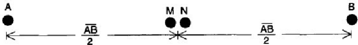
Schlumberger Electrode Array
