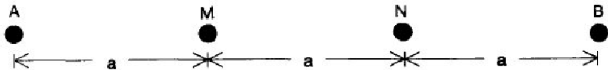
Wenner Electrode Array
