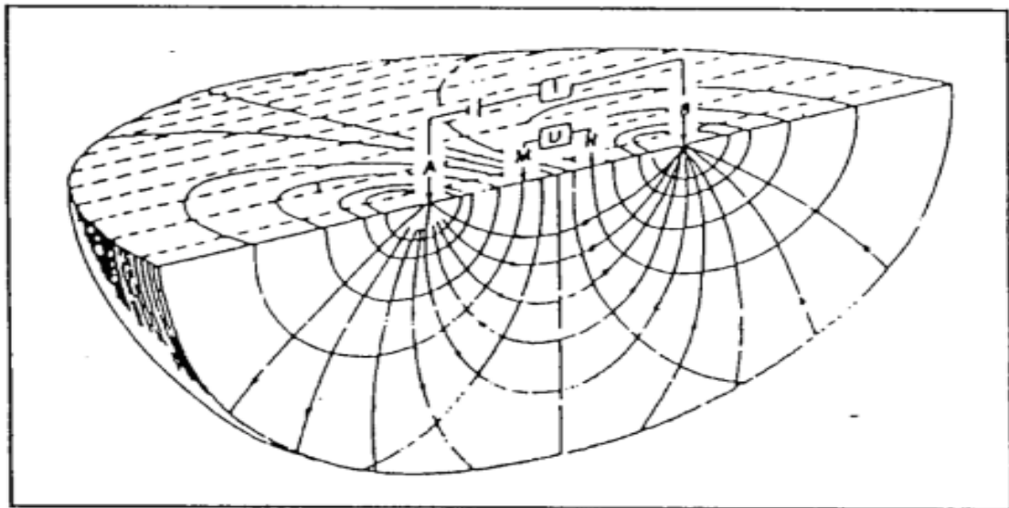
Abb. 2.3 Verlauf von Stromlinien und Äquipotentialflächen in einem geschichteten Halbraum bei einer Vierpunktanordnung (Repsold, 1991)
