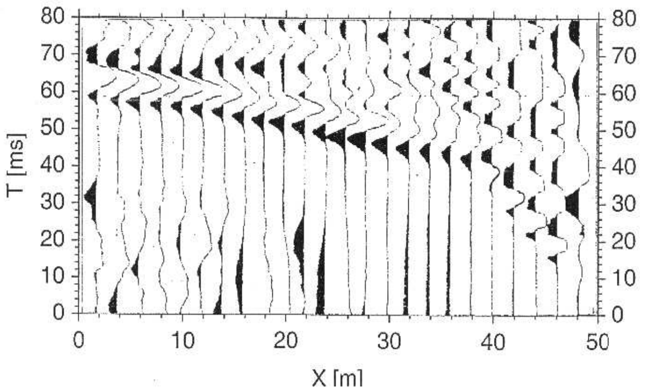
Abbildung 1: Seismogramm-Sektionen für Hinschuss A (oben) und Gegenschuss B (unten) bei einer refraktionsseismischen Feldmessung.
