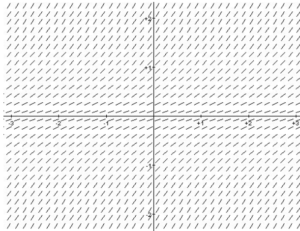
Richtungsfeld von y' = \sqrt{|y|} .
