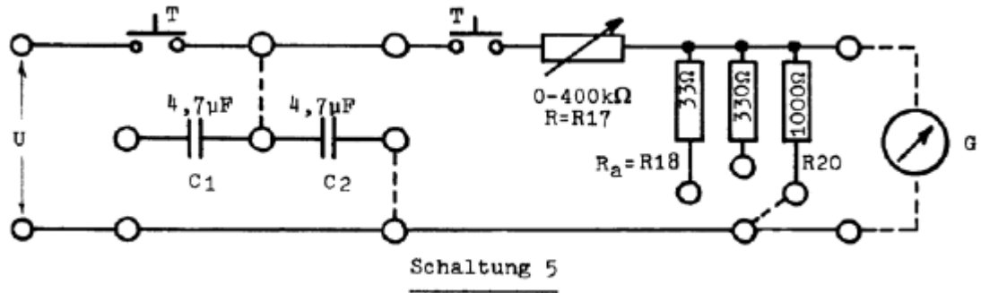
Abbildung 6: Schaltung 5
