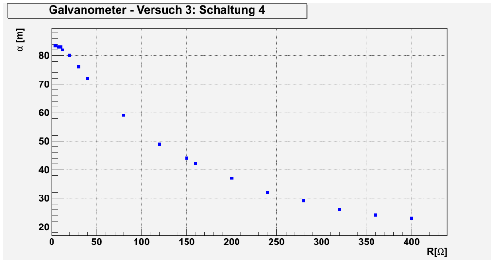
Abbildung 6: Schaltung 4
