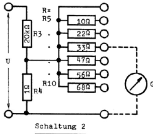
Abbildung 3: Schaltung 2
